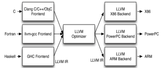
Fig. 1. LLVM Structure(2).
